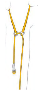
Fig. 8 - Ancoraggio passante per corda raddoppiata
