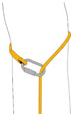
Fig. 2 - Strozzo diretto della funne
