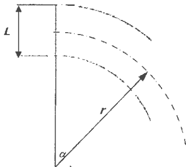
fig. 1 — rappresentazione schematica dei requisiti di curva minima
